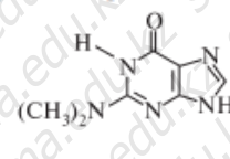
2-N,N'-диметилгуанин (m 2 G)
